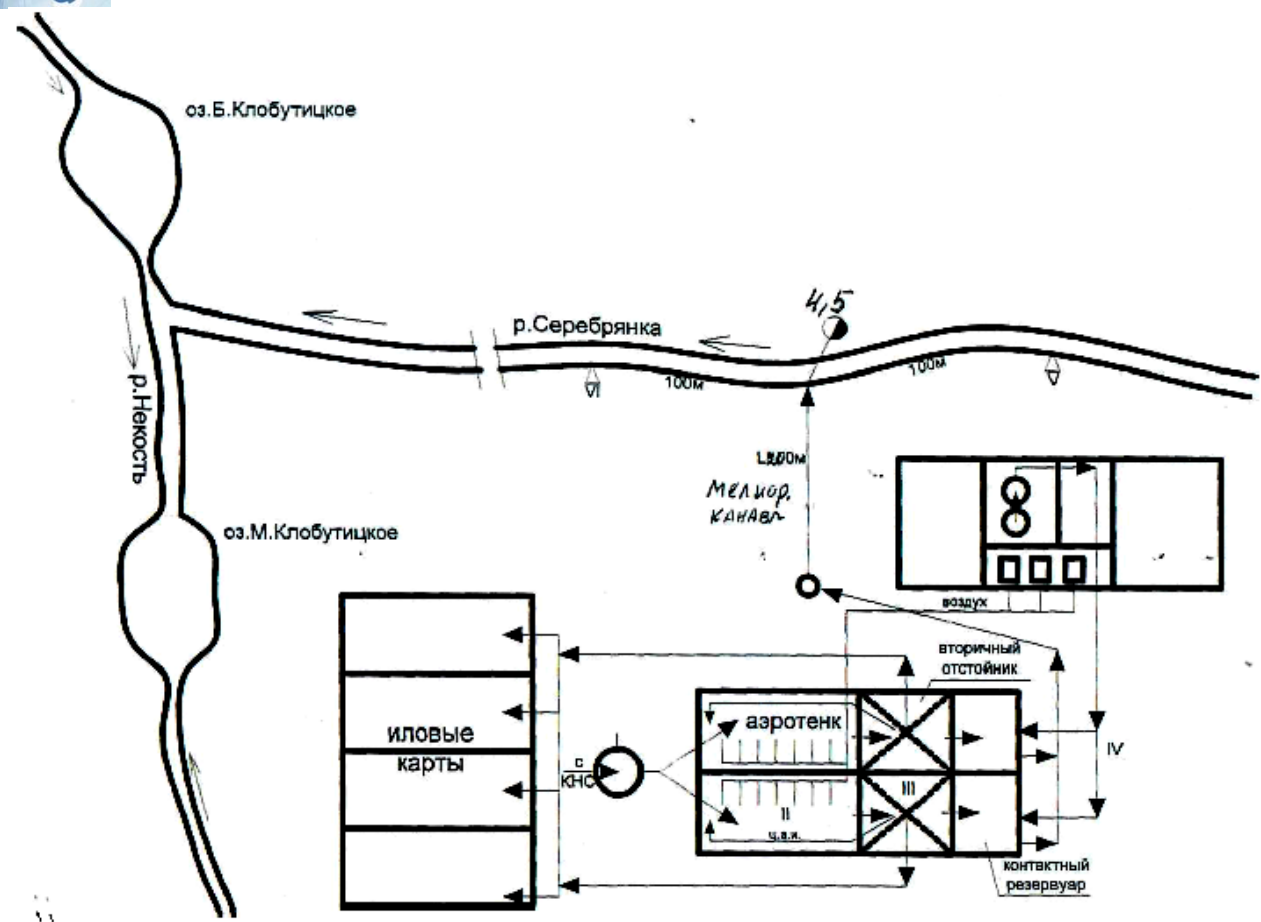
Рис. 2 План КОС пос. Серебрянский
